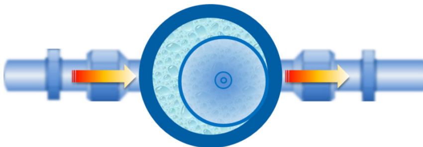
Térfogat kiszorítás elvén működő (volumetrikus)-, vízmérő
