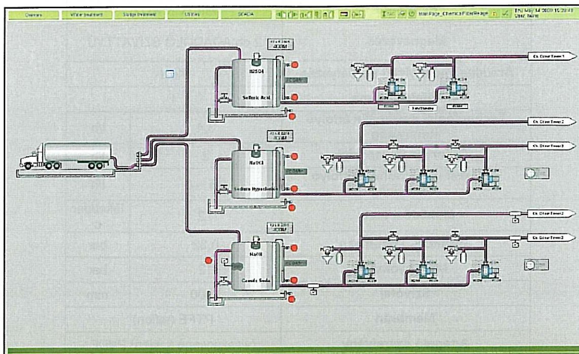
3. ábra: A kémiai szagtalanítás anyagait szállító és adagoló rendszer áttekintő rajza
