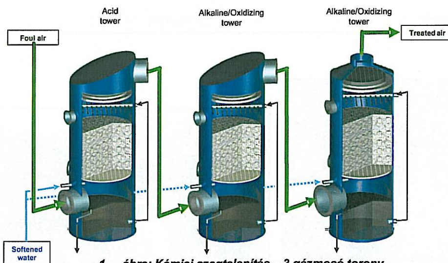
1. ábra: Kémiai szagtalanítás – 3 gázmosó torony
